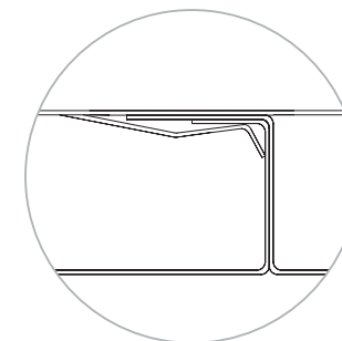
DET. A-B Clipaje Lamas Blades Linking Clipaje Lames
